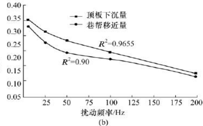
图 6 响应参数与扰动频率关系曲线
