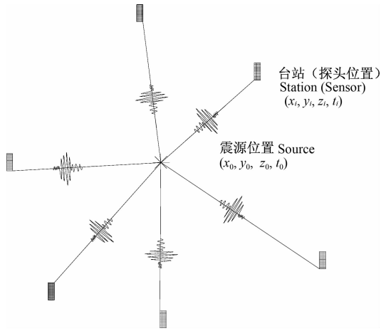
图1 矿震定位示意图
