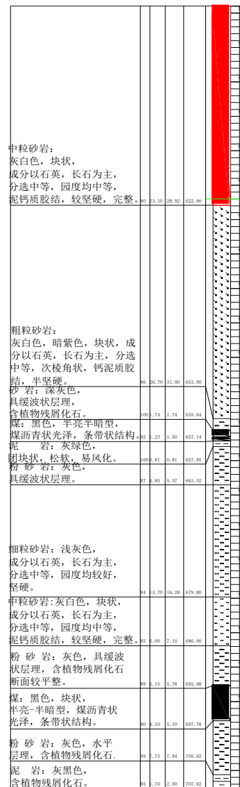
H062号钻孔
