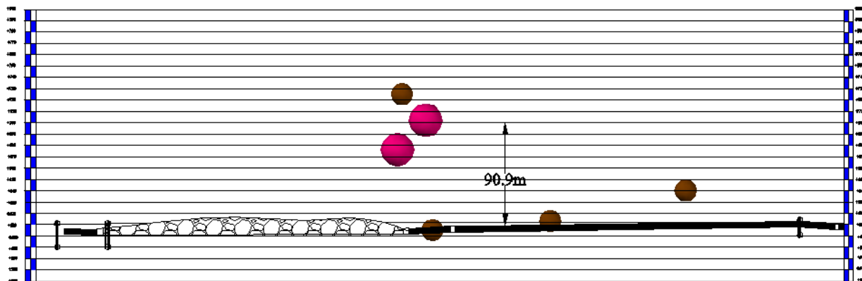
大能量事件定位剖面 ( >10^6\text{J} )
