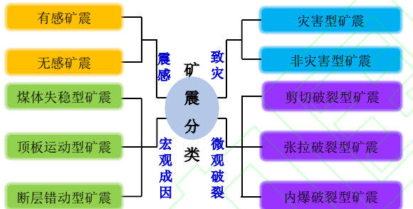
图 2 煤矿矿震分类
