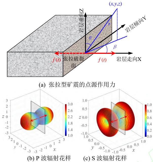
图 8 震源张拉破裂示意图 Fig. 8 Source tension rupture
