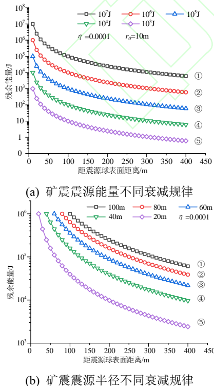
图 12 不同因素对震动波能量衰减的影响
