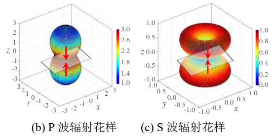
图 9 震源内爆破裂示意图
