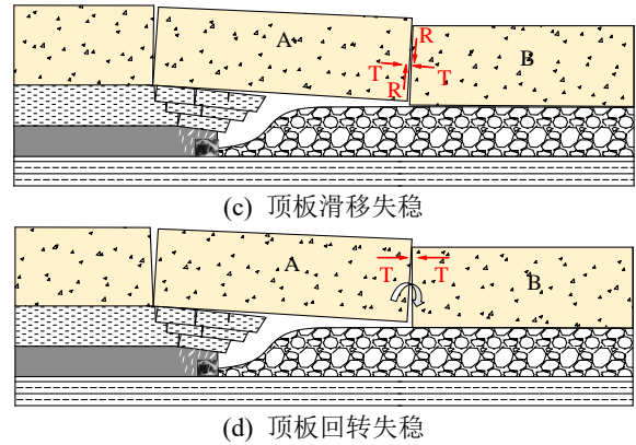
图6 顶板破断运动诱发矿震的概念模型
