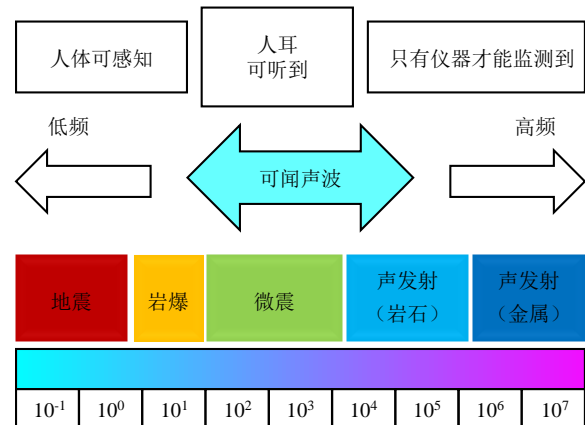
图 1 震动事件频谱 [42]
