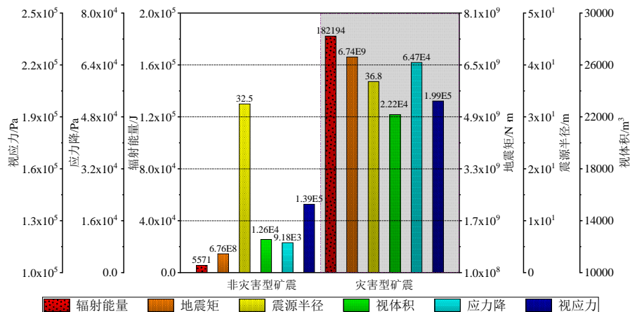
图 11 矿震震源力学参量
