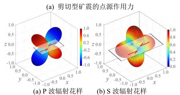
图 10 震源剪切破裂示意图
